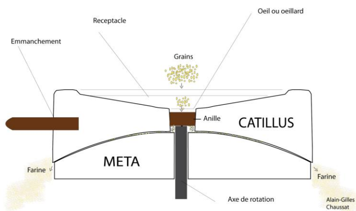
Meule romaine. La partie basse est appelée dormante, ou gisante.
