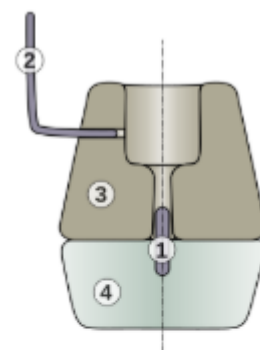
Coupe transversale d'un moulin à bras de type celtique 1-Pivot 2-Levier 3-Meule courante 4-Meule gisante.
